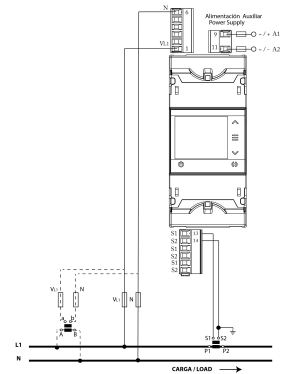
2W: 1Ph+N
