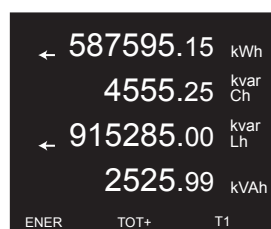
Figura 28: Valores de energía superiores a los dígitos del display.
