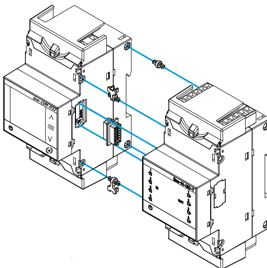
Figura 9: Instalación paso 2.
