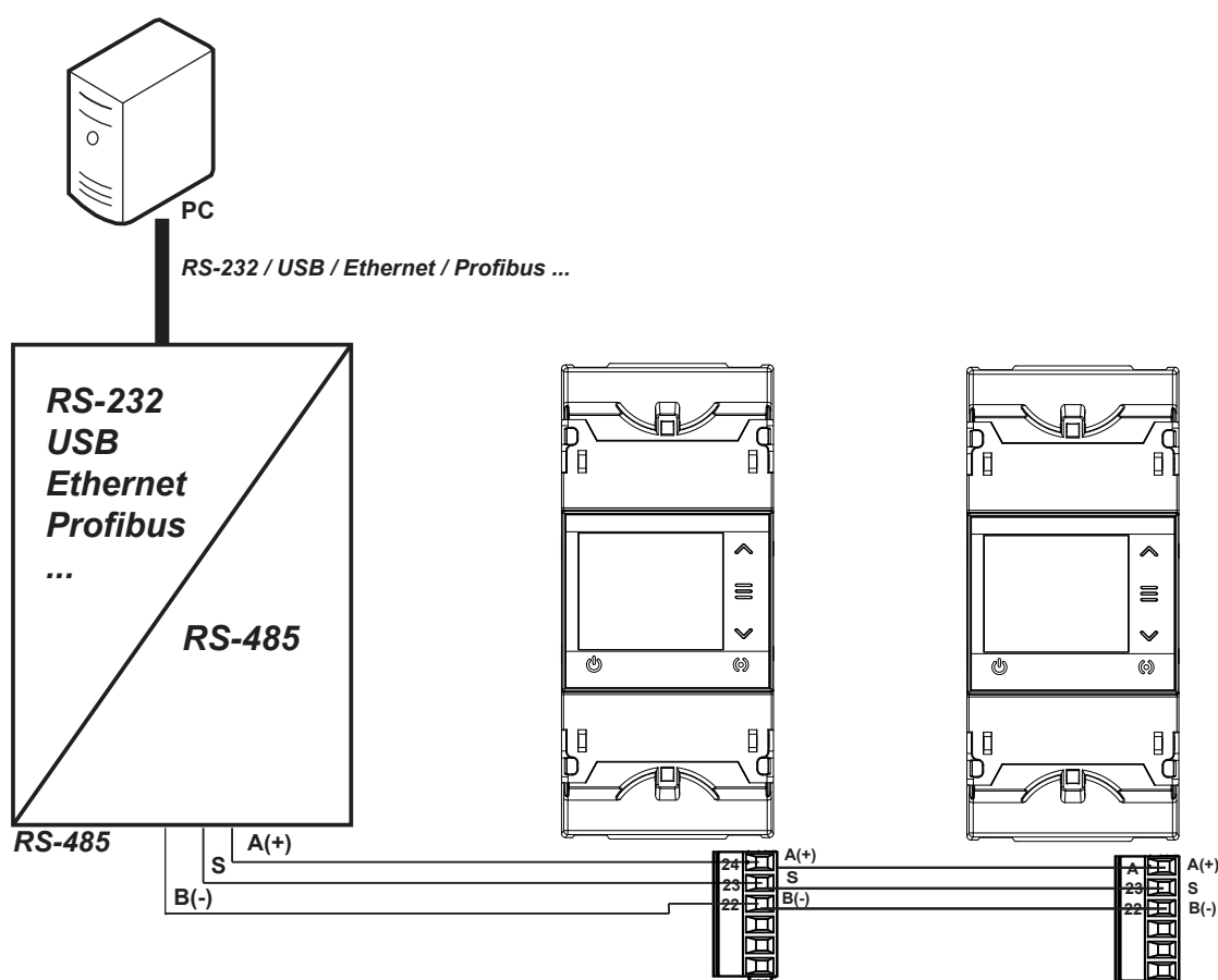
Figura 31: Esquema de conexionado RS-485.
