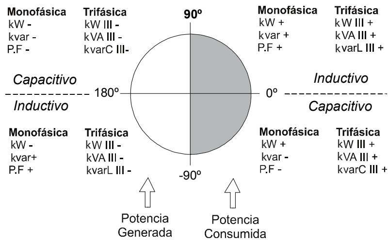
Figura 25: Convenio de medida CIRCUITOR.
