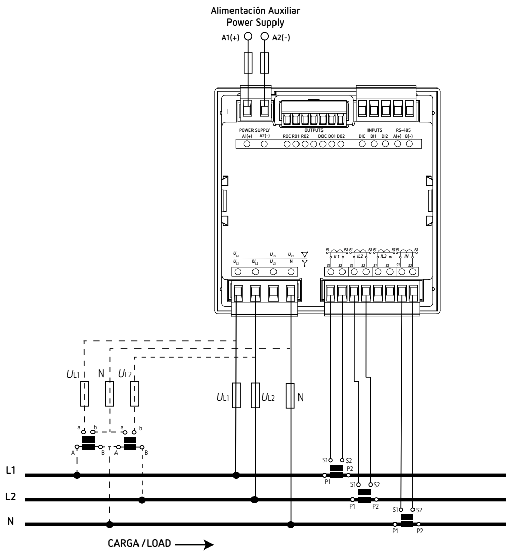
Figura 13: Medida bifásica con conexión a 3 hilos (CVM-C11-ITF-IN-xxx-ICT2).
