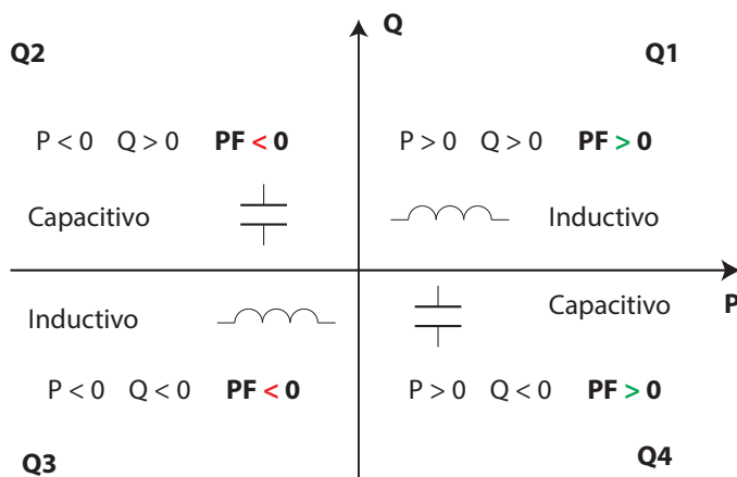
Figura 26: Convenio de medida IEC 61557-12.
