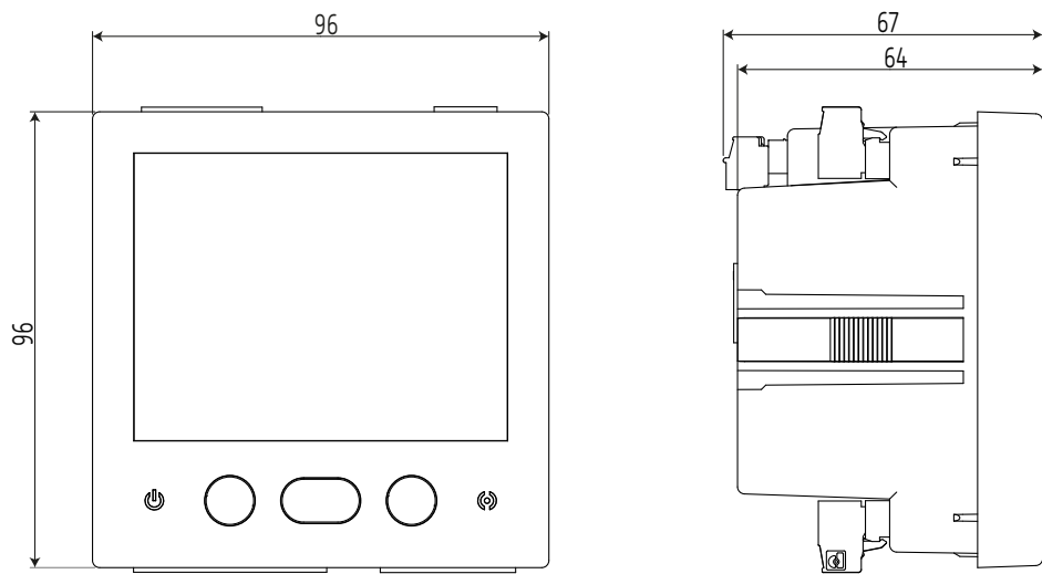
Figura 41: Dimensiones del CVM-C11.
