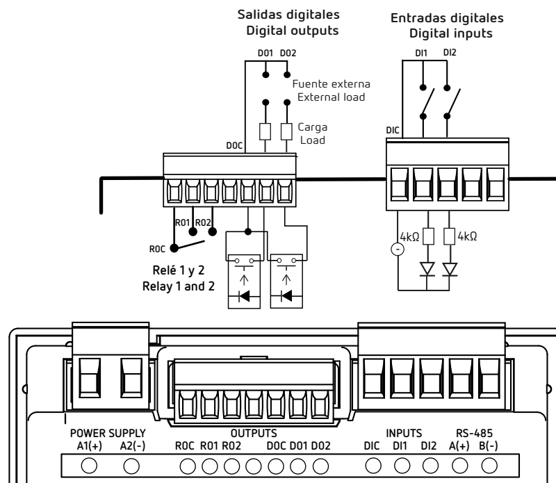
Figura 35: Relés, Salidas digitales y Entradas digitales.
