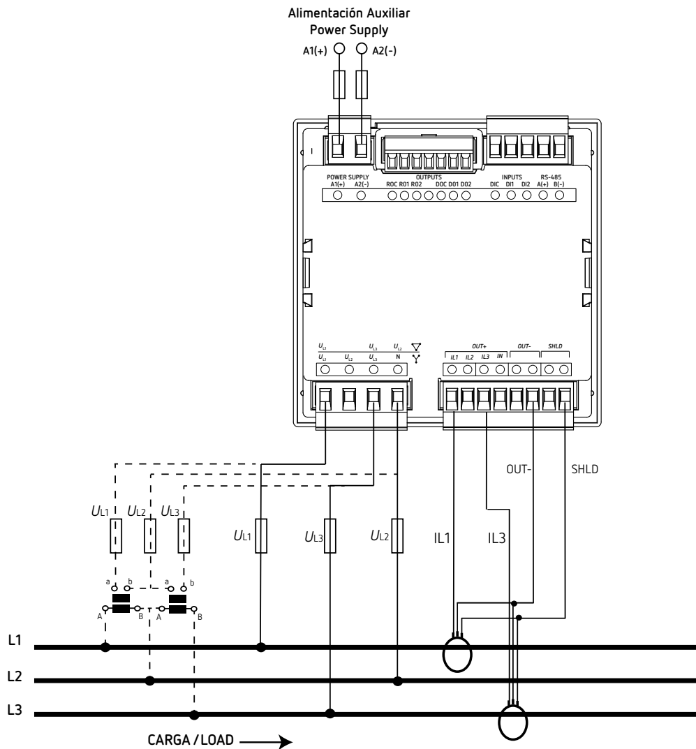
Figura 12: Medida trifásica con conexión a 3 hilos y transformadores en conexión ARON (CVM-C11-FLEX-IN-485-ICT2).
