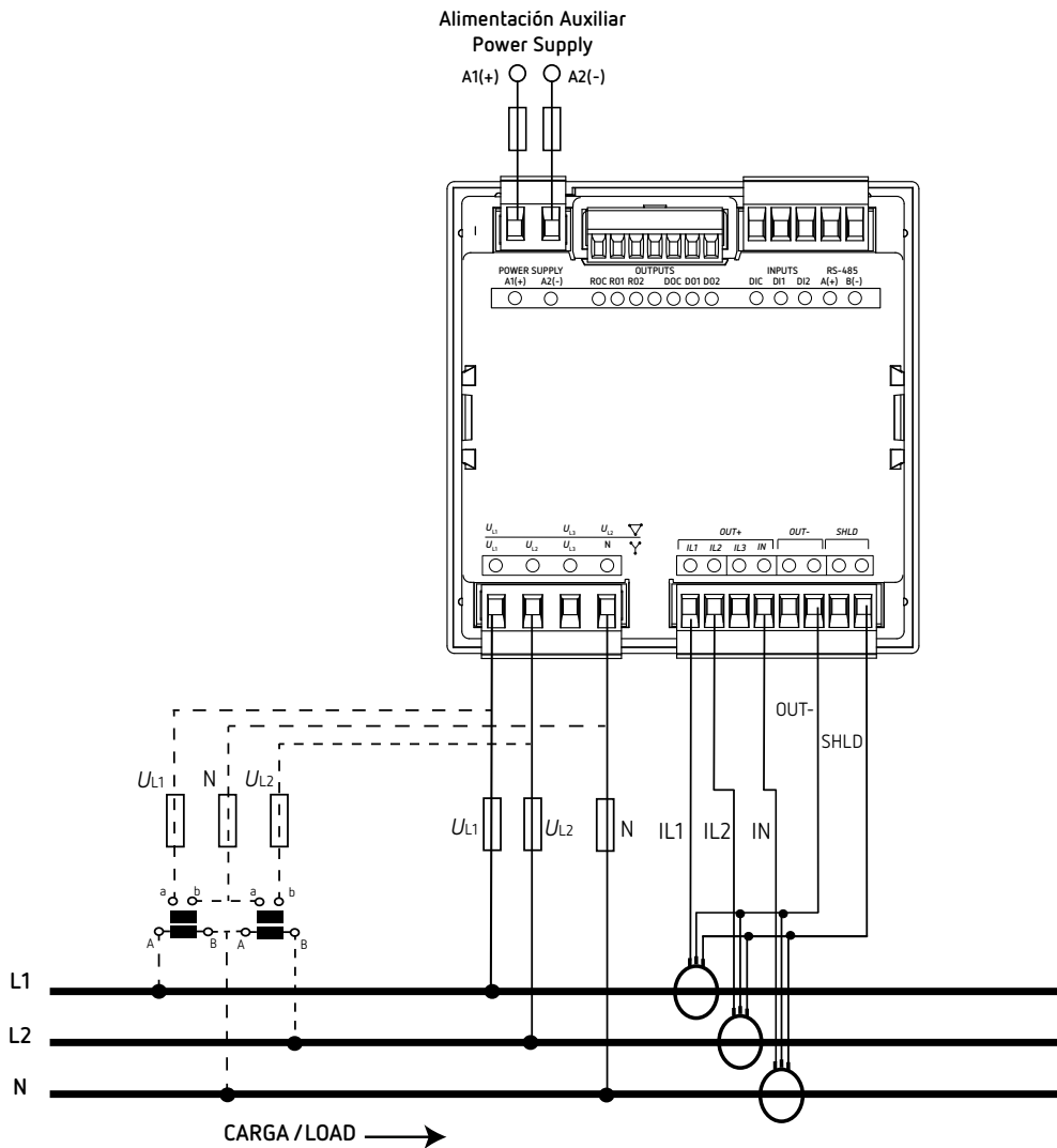
Figura 15: Medida bifásica con conexión a 3 hilos (CVM-C11-FLEX-IN-485-ICT2).
