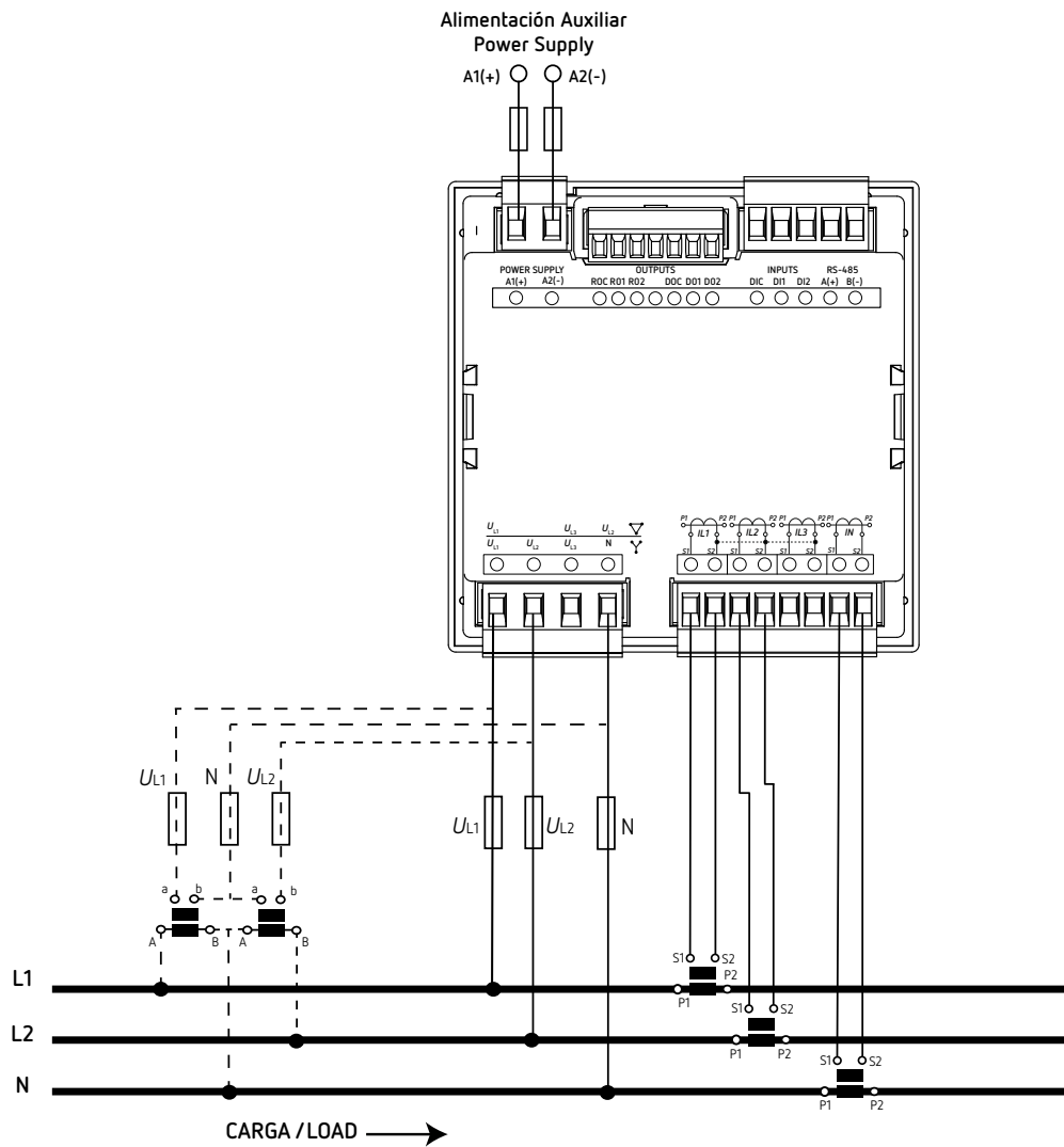
Figura 14: Medida bifásica con conexión a 3 hilos (CVM-C11-MC-IN-485-ICT2).
