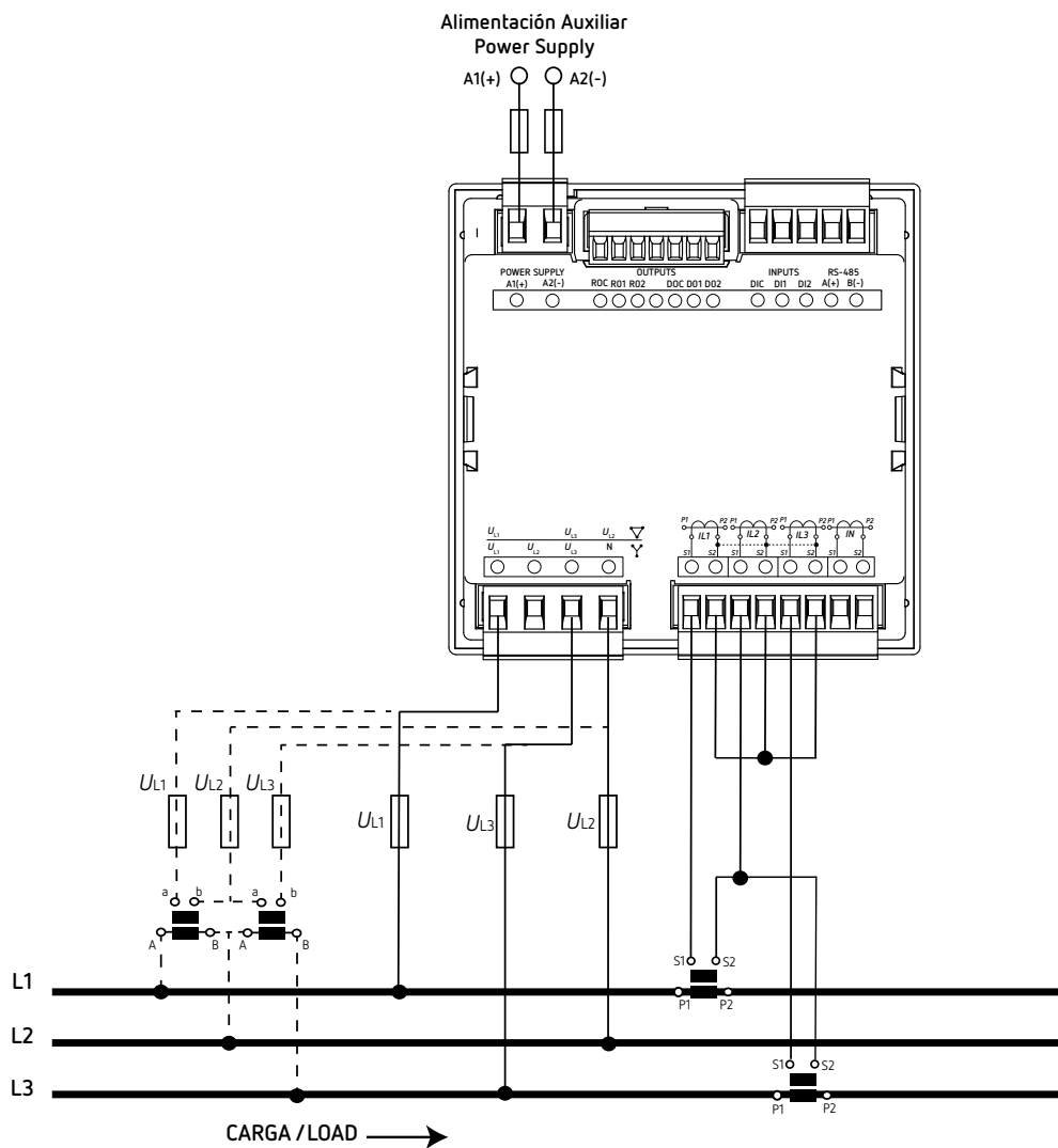
Figura 11: Medida trifásica con conexión a 3 hilos y transformadores en conexión ARON (CVM-C11-MC-IN-485-ICT2).
