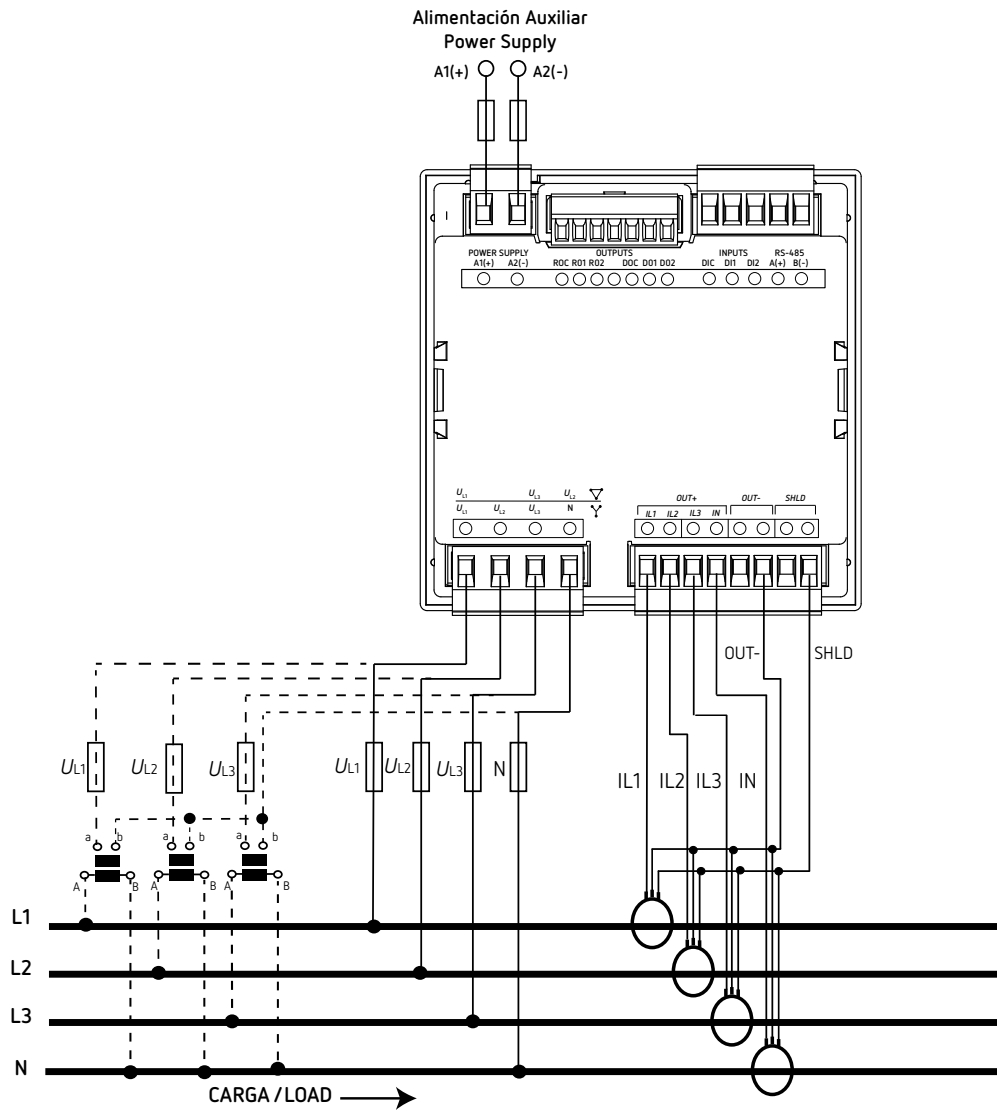
Figura 6: Medida trifásica con conexión a 4 hilos (CVM-C11-FLEX-IN-485-ICT2).
