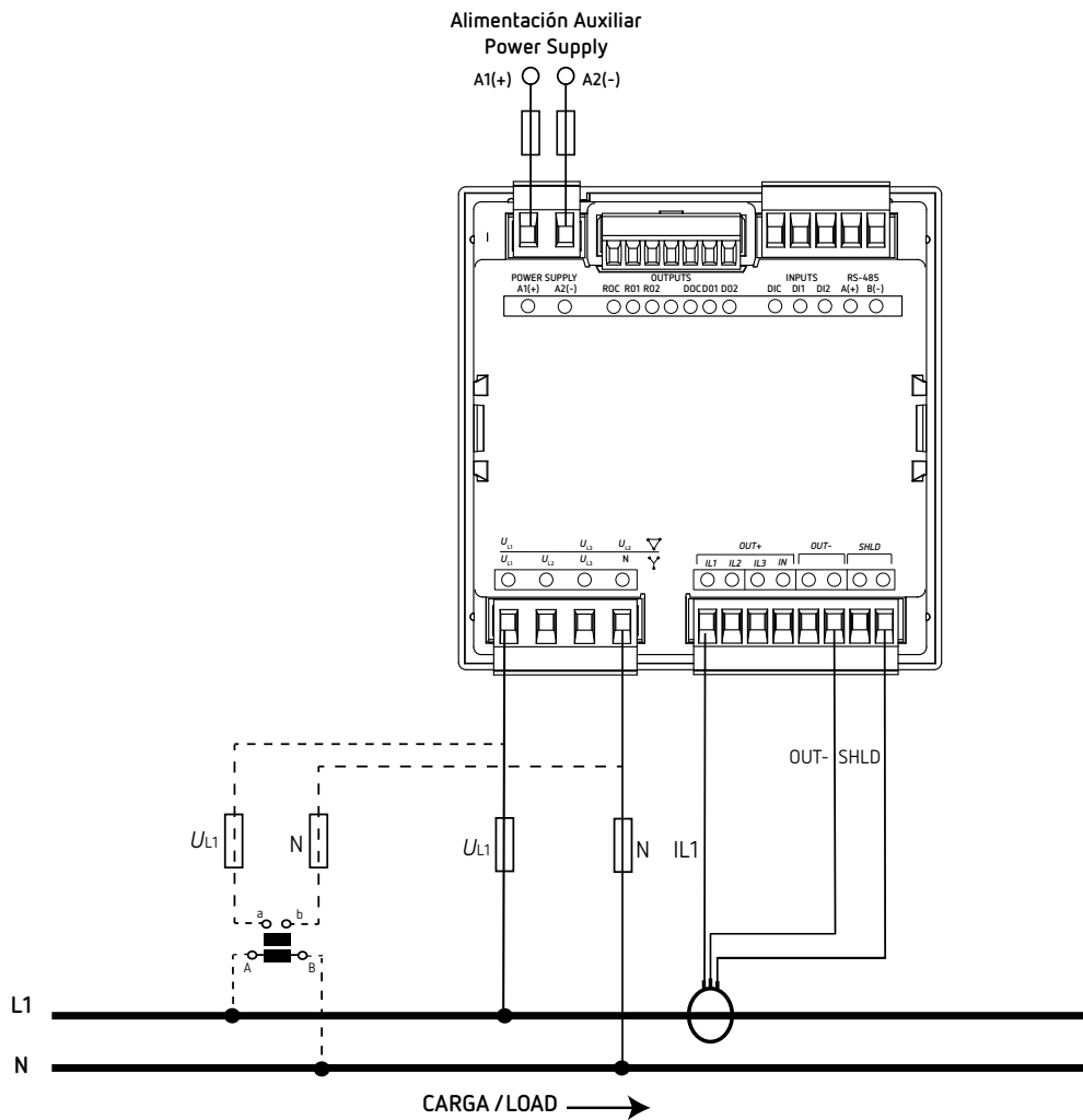
Figura 21: Medida monofásica fase a neutro de 2 hilos (CVM-C11-FLEX-IN-485-ICT2).
