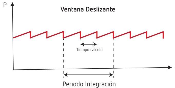
Figura 29:Ventana Deslizante.
