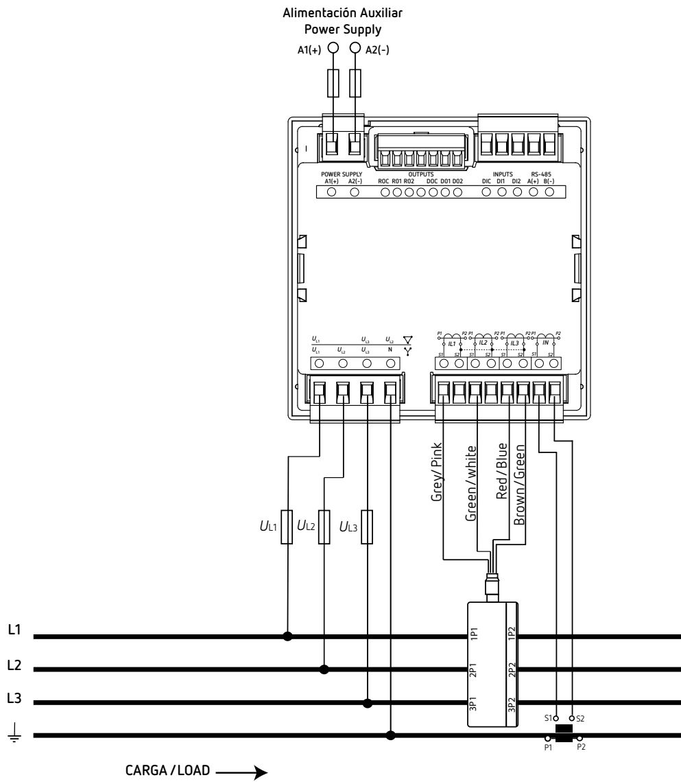
Figura 23: Medida trifásica con conexión a 3 hilos y tierra (CVM-C11-MC-IN-485-ICT2).
