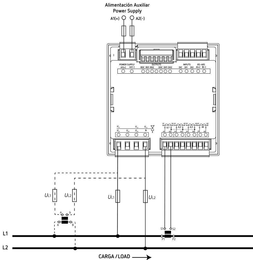
Figura 17: Medida monofásica fase a fase de 2 hilos (CVM-C11-MC-IN-485-ICT2).
