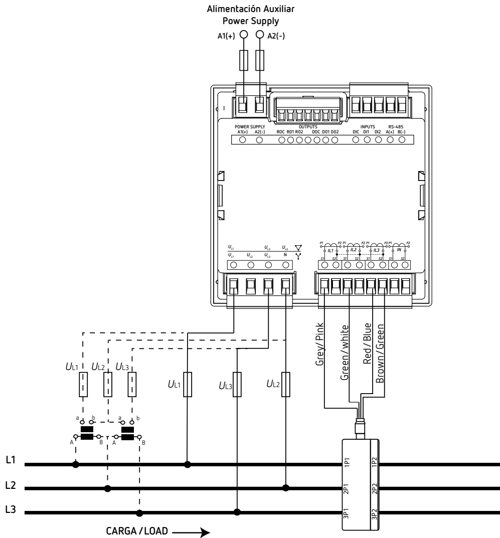
Figura 8: Medida trifásica con conexión a 3 hilos (CVM-C11-MC-IN-485-ICT2).
