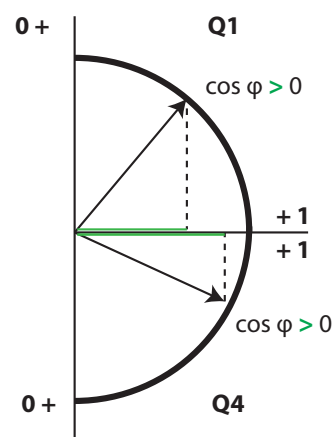
Figura 26: Convenio de medida IEC 61557-12.
