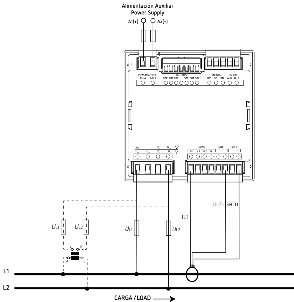
Figura 18: Medida monofásica fase a fase de 2 hilos (CVM-C11-FLEX-IN-485-ICT2).
