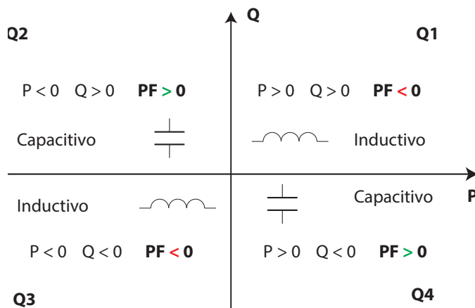
Figura 27: Convenio de medida IEEE 1459.
