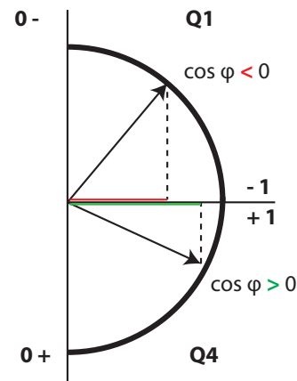
Figura 27: Convenio de medida IEEE 1459.
