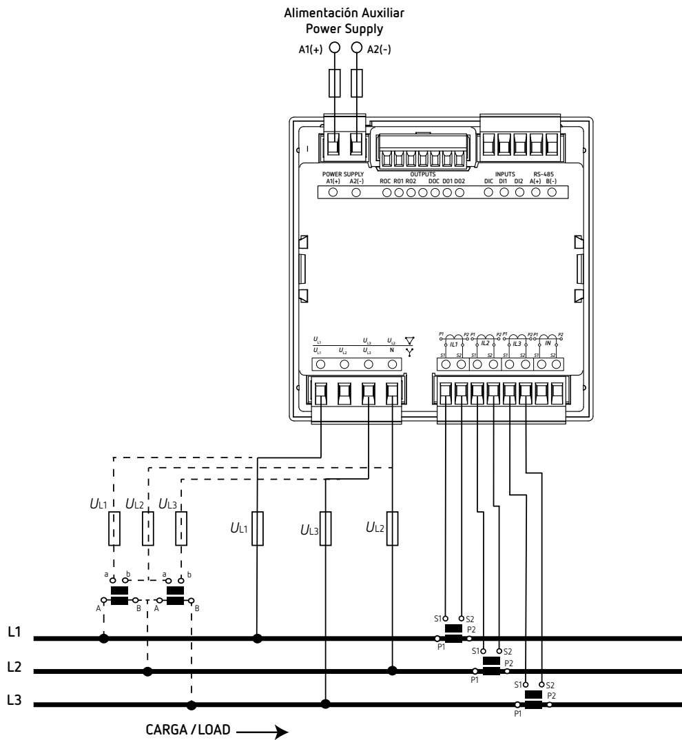
Figura 7: Medida trifásica con conexión a 3 hilos (CVM-C11-ITF-IN-xxx-ICT2).
