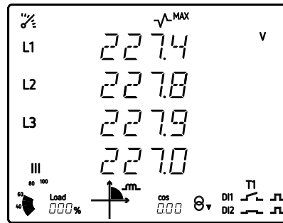
Figura 36: Pantalla del perfil analizador visualizando los valores máximos.
