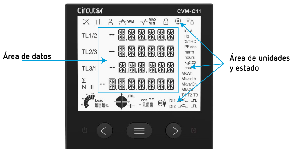
Figura 30: Áreas del display del CVM-C11.
