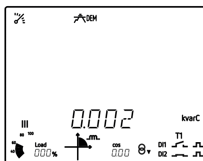
Figura 37: Pantalla del perfil analizador visualizando los valores de máxima demanda.
