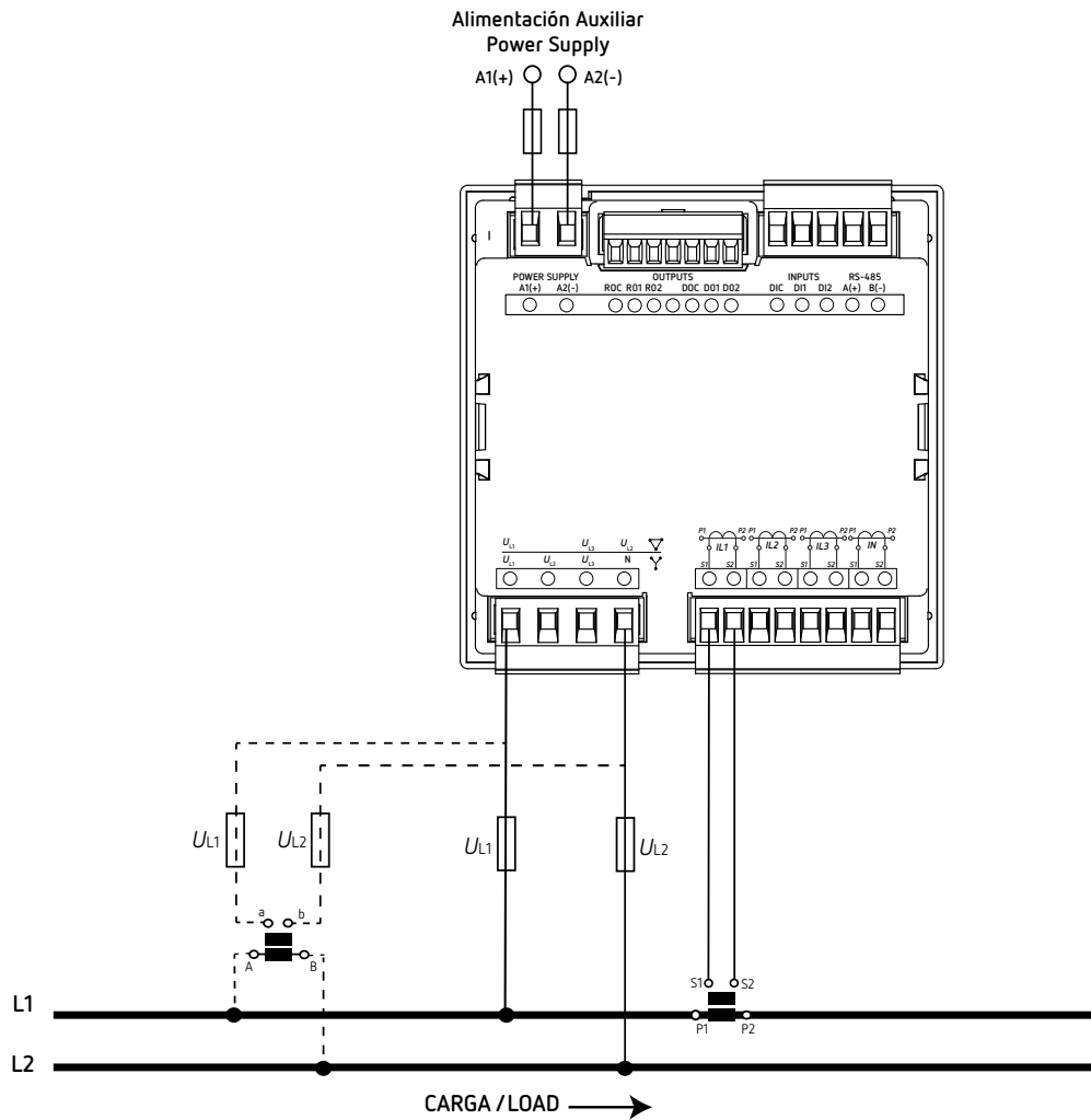
Figura 16: Medida monofásica fase a fase de 2 hilos (CVM-C11-ITF-IN-xxx-ICT2).
