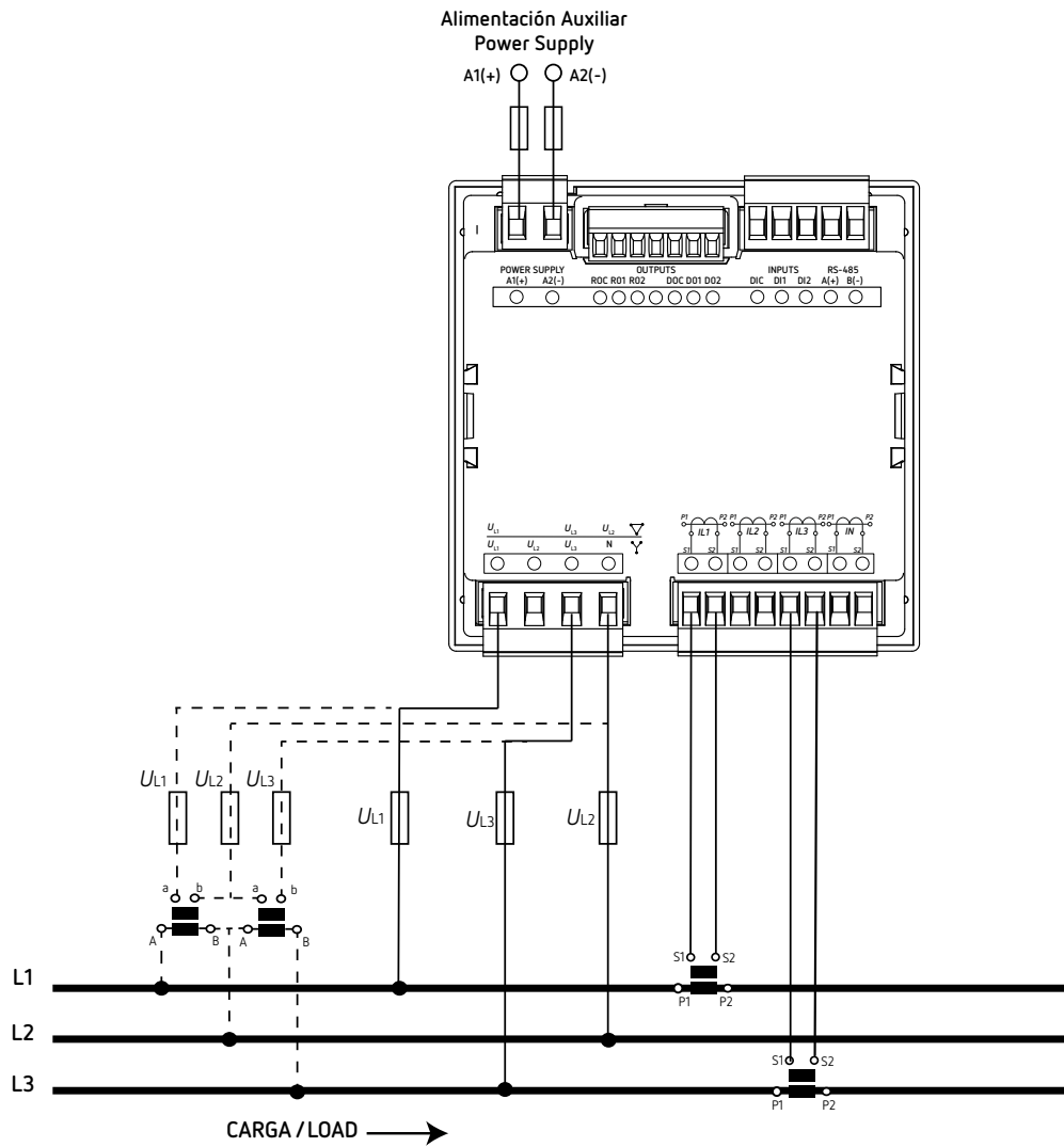
Figura 10: Medida trifásica con conexión a 3 hilos y transformadores en conexión ARON (CVM-C11-ITF-IN-xxx-ICT2).
