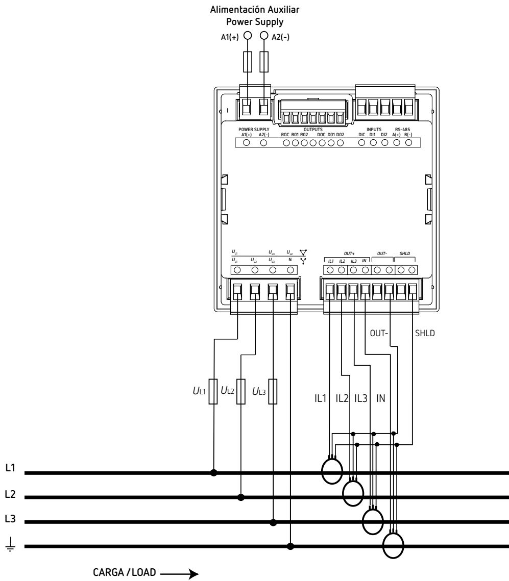
Figura 24: Medida trifásica con conexión a 3 hilos y tierra (CVM-C11-FLEX-IN-485-ICT2).
