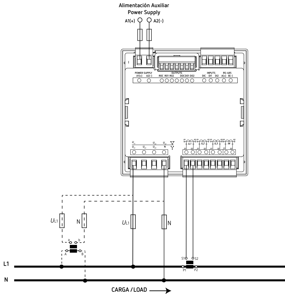
Figura 19: Medida monofásica fase a neutro de 2 hilos (CVM-C11-ITF-IN-xxx-ICT2).
