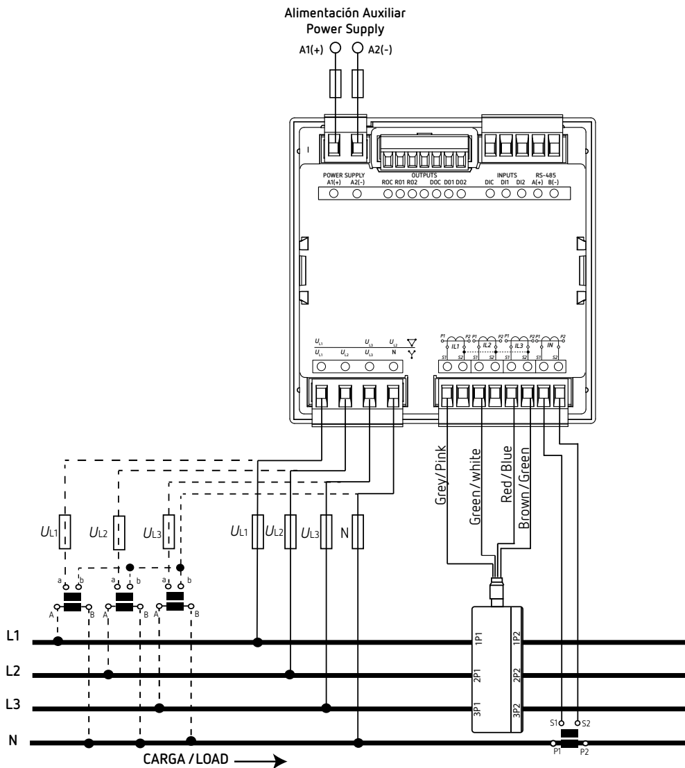
Figura 5: Medida trifásica con conexión a 4 hilos (CVM-C11-MC-IN-485-ICT2).
