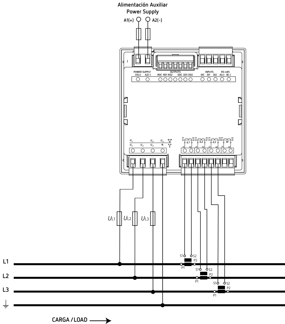
Figura 22: Medida trifásica con conexión a 3 hilos y tierra (CVM-C11-ITF-IN-xxx-ICT2).
