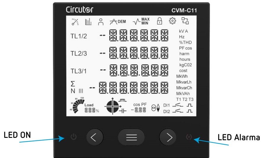
Figura 34: Indicadores LED del CVM-C11.
