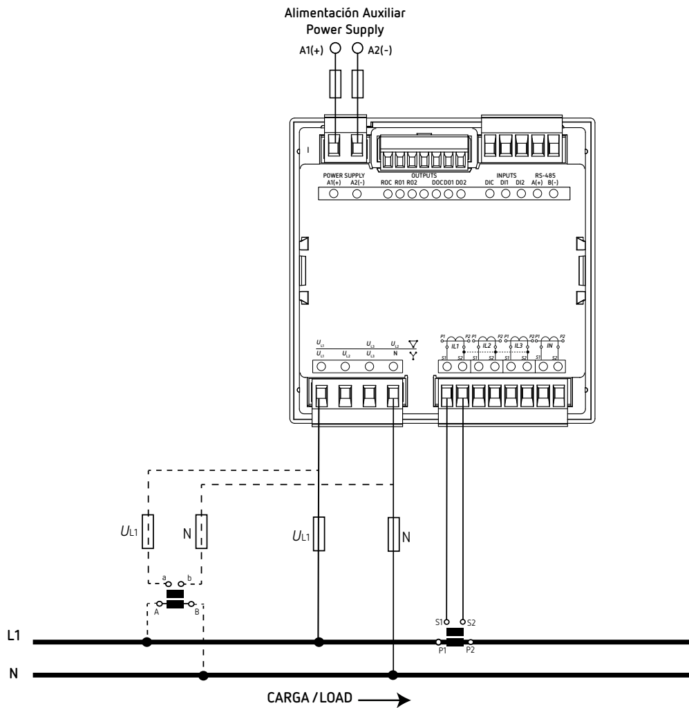
Figura 20: Medida monofásica fase a neutro de 2 hilos (CVM-C11-MC-IN-485-ICT2).
