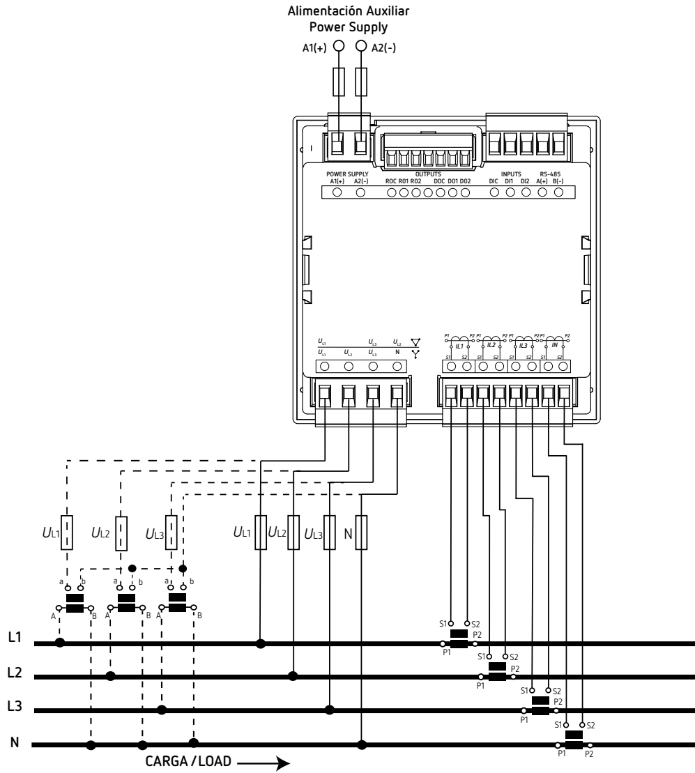
Figura 4: Medida trifásica con conexión a 4 hilos (CVM-C11-ITF-IN-xxx-ICT2).
