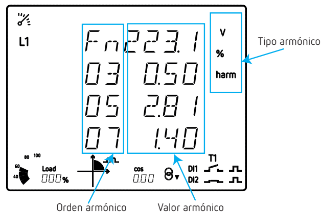
Figura 39: Pantalla de los armónicos del CVM-C11.
