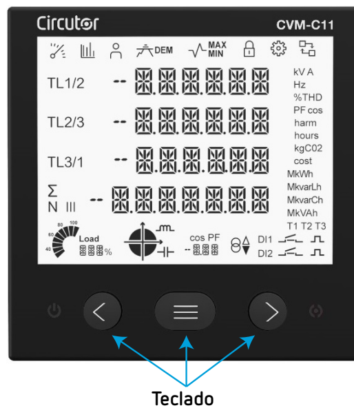
Figura 33: Teclado del CVM-C11.
