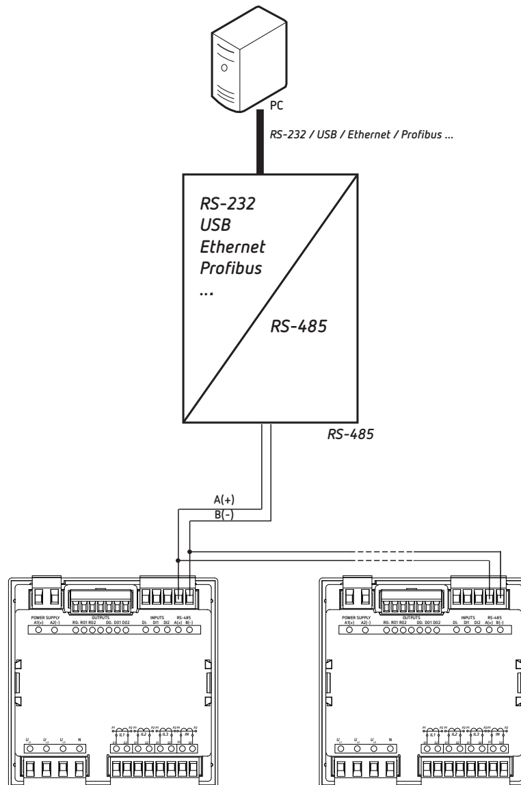
Figura 40: Esquema de conexionado RS-485.
