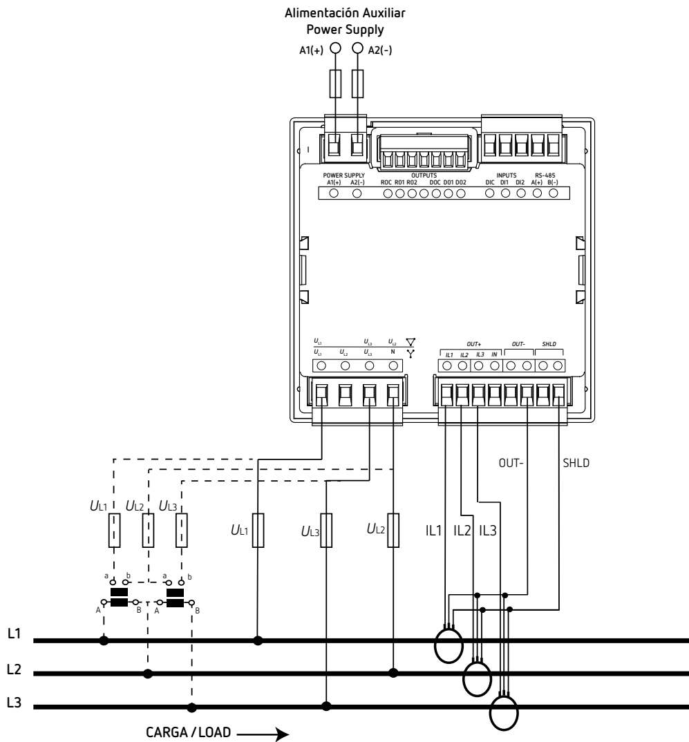
Figura 9: Medida trifásica con conexión a 3 hilos (CVM-C11-FLEX-IN-485-ICT2).
